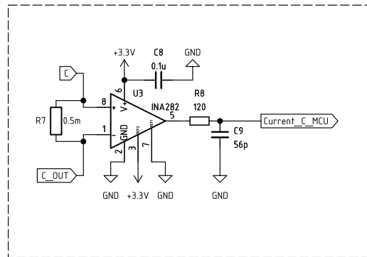
Измерение тока С
