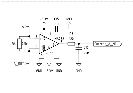
Измерение тока А
