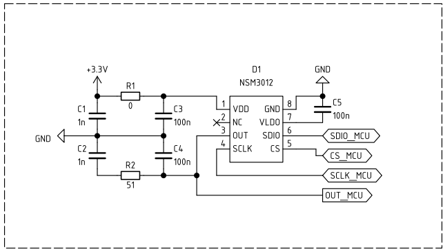
Датчик положения
