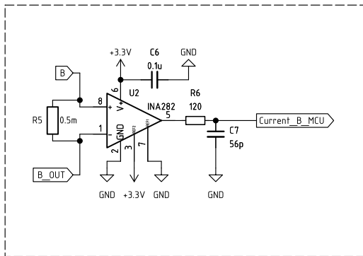
Измерение тока В
